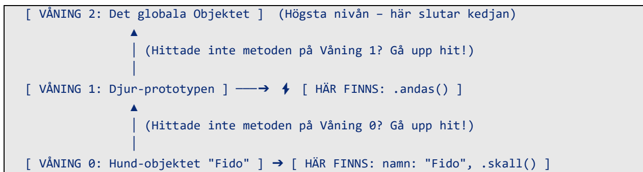
Bild 1 JavaScript letar uppåt i en kedja av objekt tills det hittar metoden.
